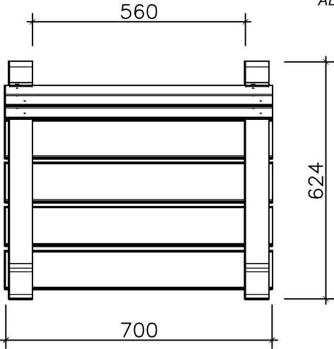
PLANTA Top View
