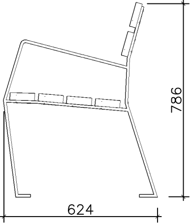
ALÇADO LATERAL Side View
