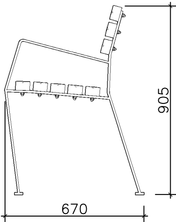
ALÇADO LATERAL Side View
